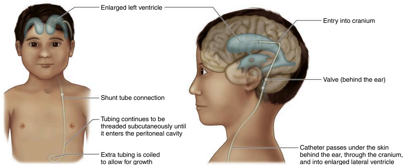
FIG. 39.4 Ventriculoperitoneal shunt.
