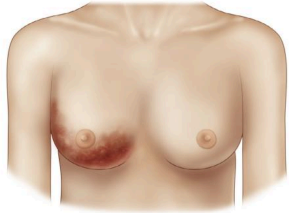
FIG. 27.3 Mastitis.
